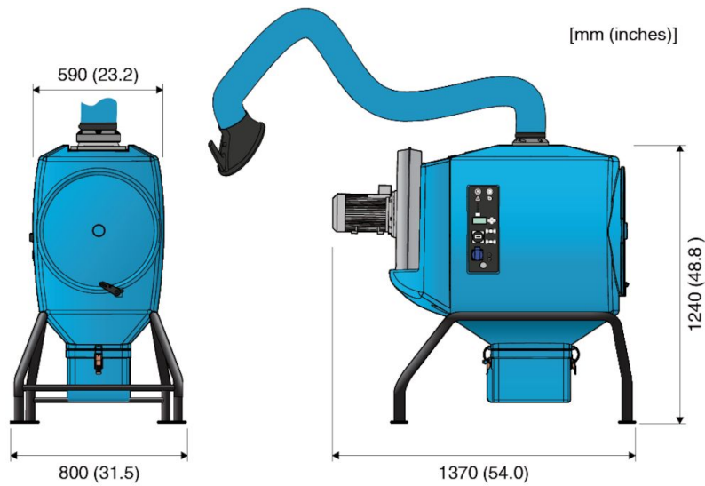
Na podlahe instalovaný FilterBox 12A
