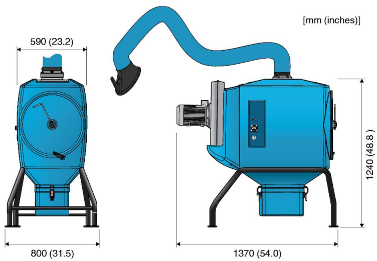
Na podlahe instalovaný FilterBox 12M
